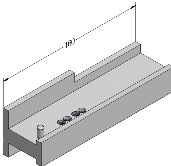
Шаблон импоста
